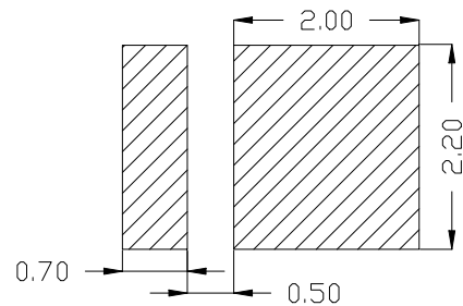
建议焊盘
